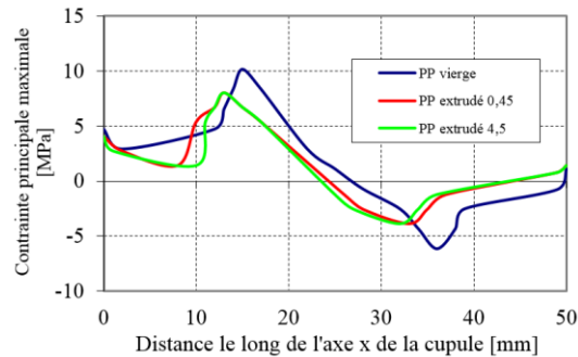
Figure 10. Evolution des contraintes principales maximales le long de l'axe x
