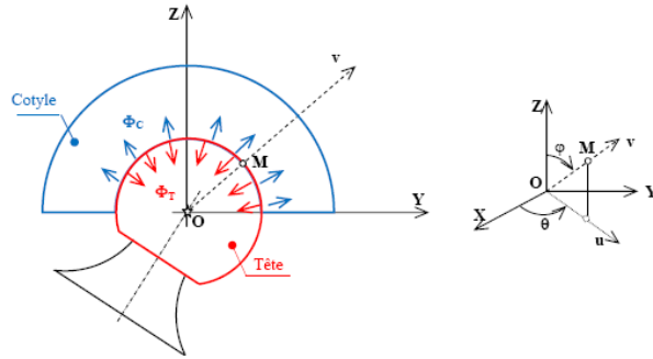
Figure 4. Modélisation du couple cupule tête fémorale
