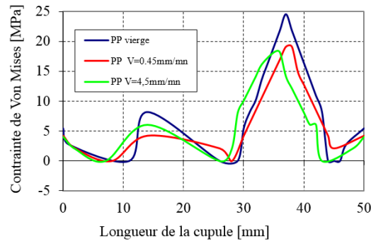
Figure 7. Evolution des contraintes équivalentes de Von Mises le long de l’axe x
