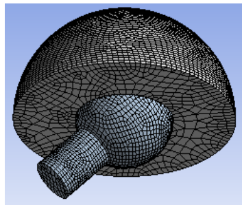
Figure 5. La discrétisation du modèle en éléments finis
