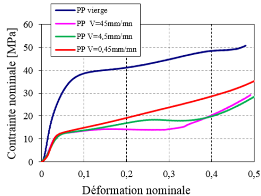
Figure 3. Evolutions de la contrainte en fonction de la déformation des échantillons de PP vierge et du PP extrudé à différentes vitesses d'extrusion [2,3]
