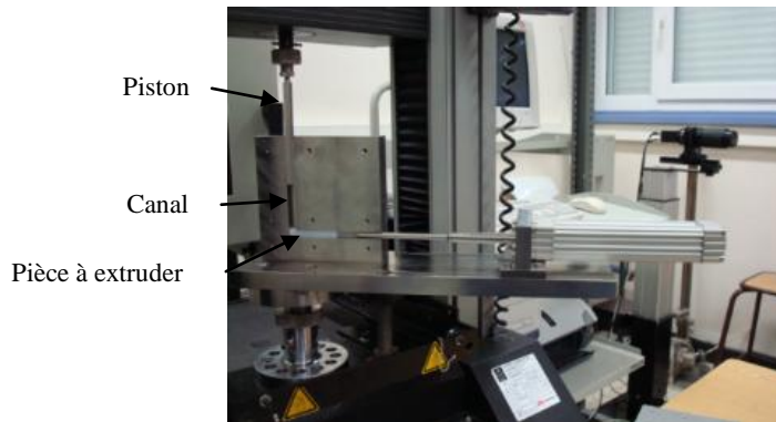
Figure 2. Dispositif expérimental d'extrusion angulaire à section constante [2,3]
