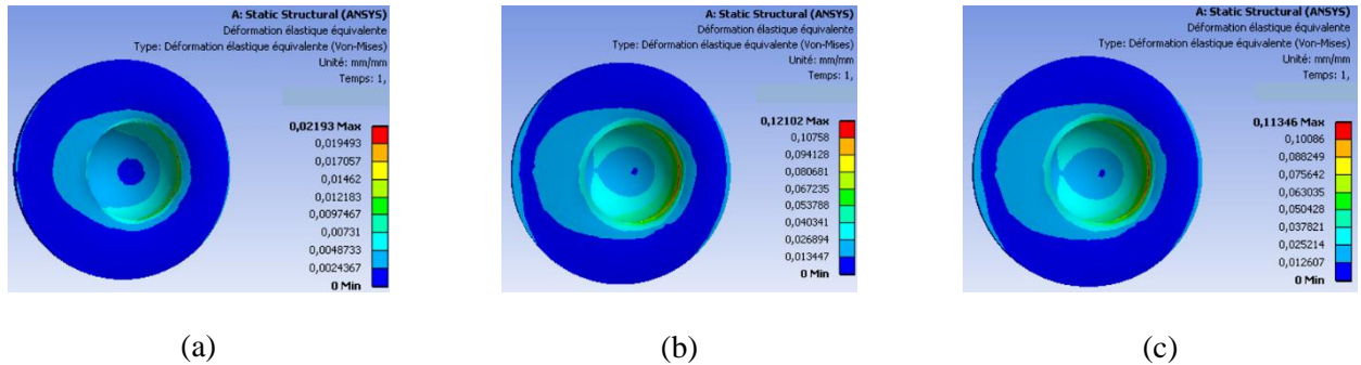
Figure 8. déformation élastique équivalente d'une coupule en service fabriquée en : (a) PP vierge, (b) PP extrudé à 0,45 mm/mm et (c) PP extrudé à 0,45 mm/mm
