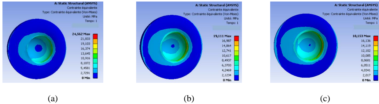
Figure 6. Contraintes équivalente de Von Mises d’une cupule en service fabriquée en :
